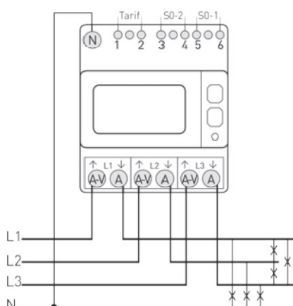
3 PHASEN - 4 LEITER
