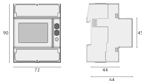
Abmessungen (mm):
