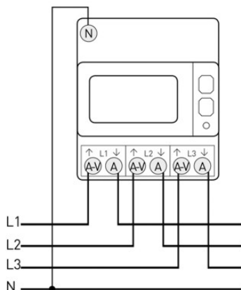
3 Phasen - 4 Leiter
